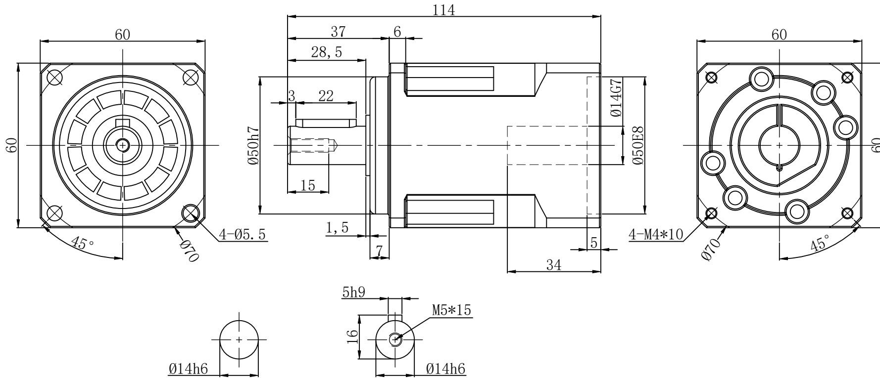
轴型式 S1
